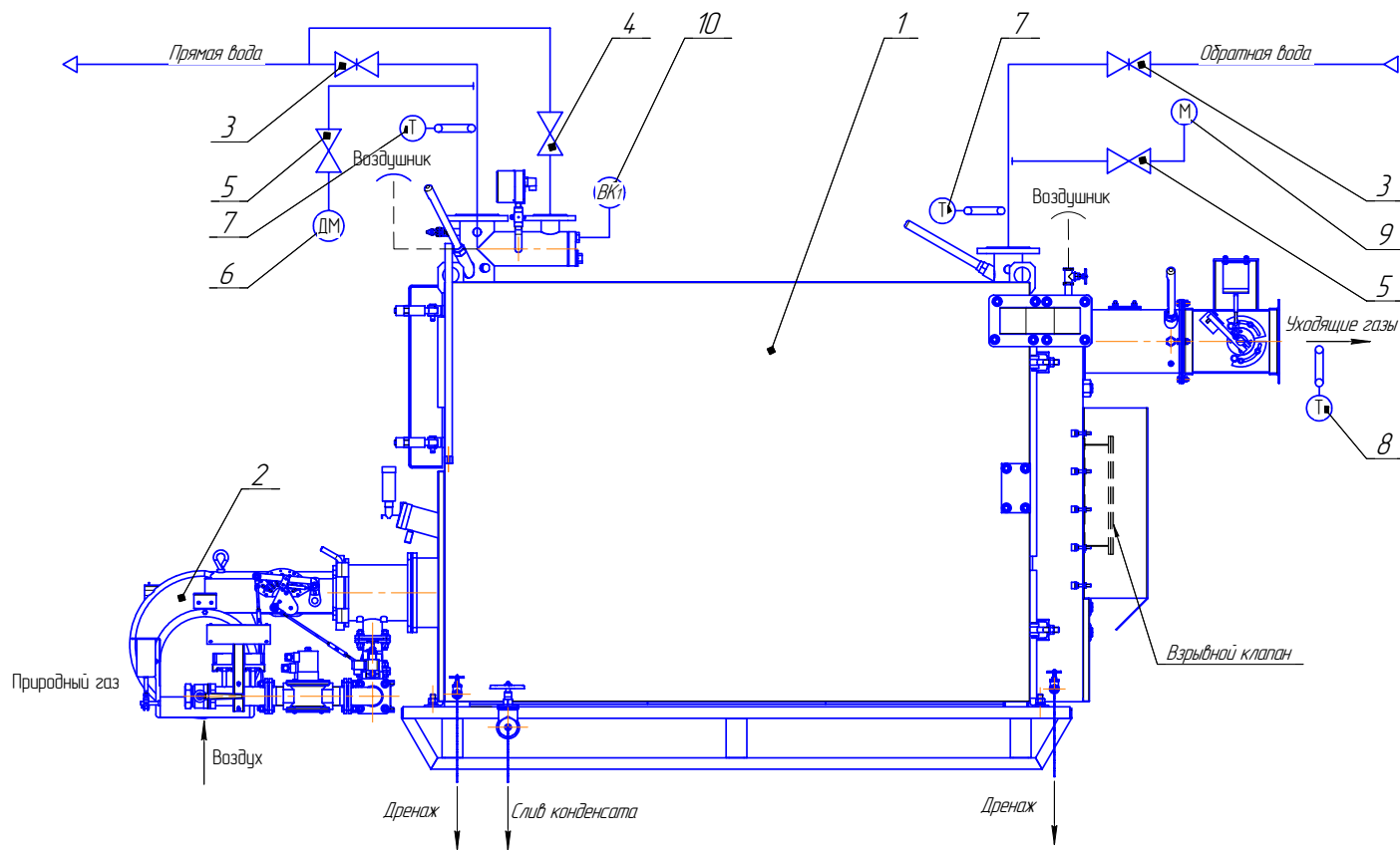
РИС. 1 СХЕМА ФУНКЦИОНАЛЬНАЯ КОТЛА КСВа-0,25
