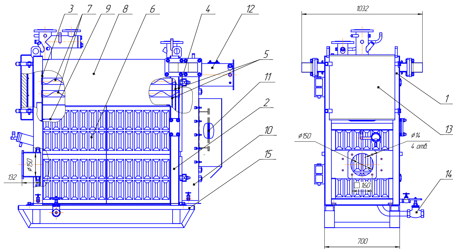
РИС. 2 КОТЕЛ КСВа-0,25 В РАЗРЕЗЕ
