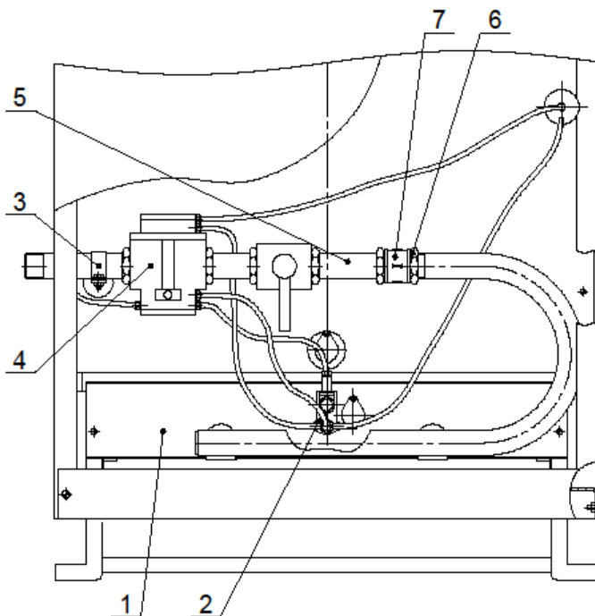
Рисунок 1.1. Котёл "Хопёр" с горелкой производства "БКМЗ" и автоматикой РГУ
